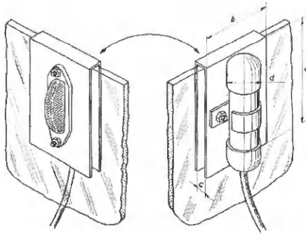
De maten a, b en d zijn afhankelijk van het toegepaste parkeerlicht-armatuur en de behuizing. De dikte van de portierraam bepaalt c.
